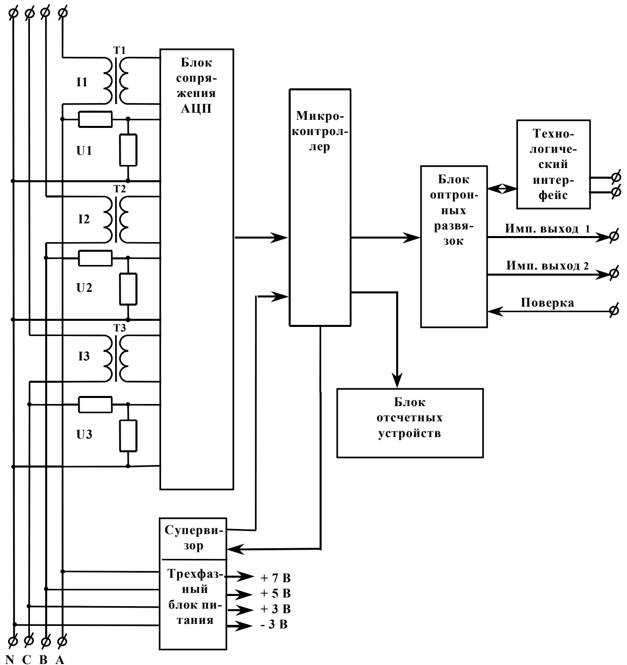
Рисунок 1 – Структурная схема устройства измерения и управления
