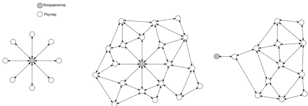
Рисунок А.1 – Топологии радиосети.
